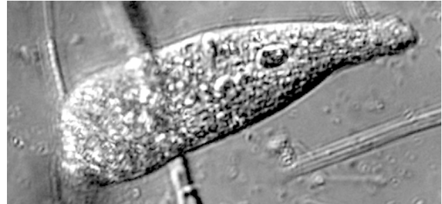
Рис. 1. Saccamoeba wakulla (x 1240)
