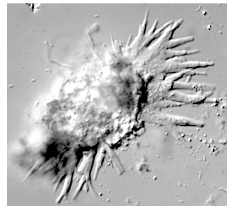
Рис. 3. Rhizamoeba sp. (2) (x 1240)
