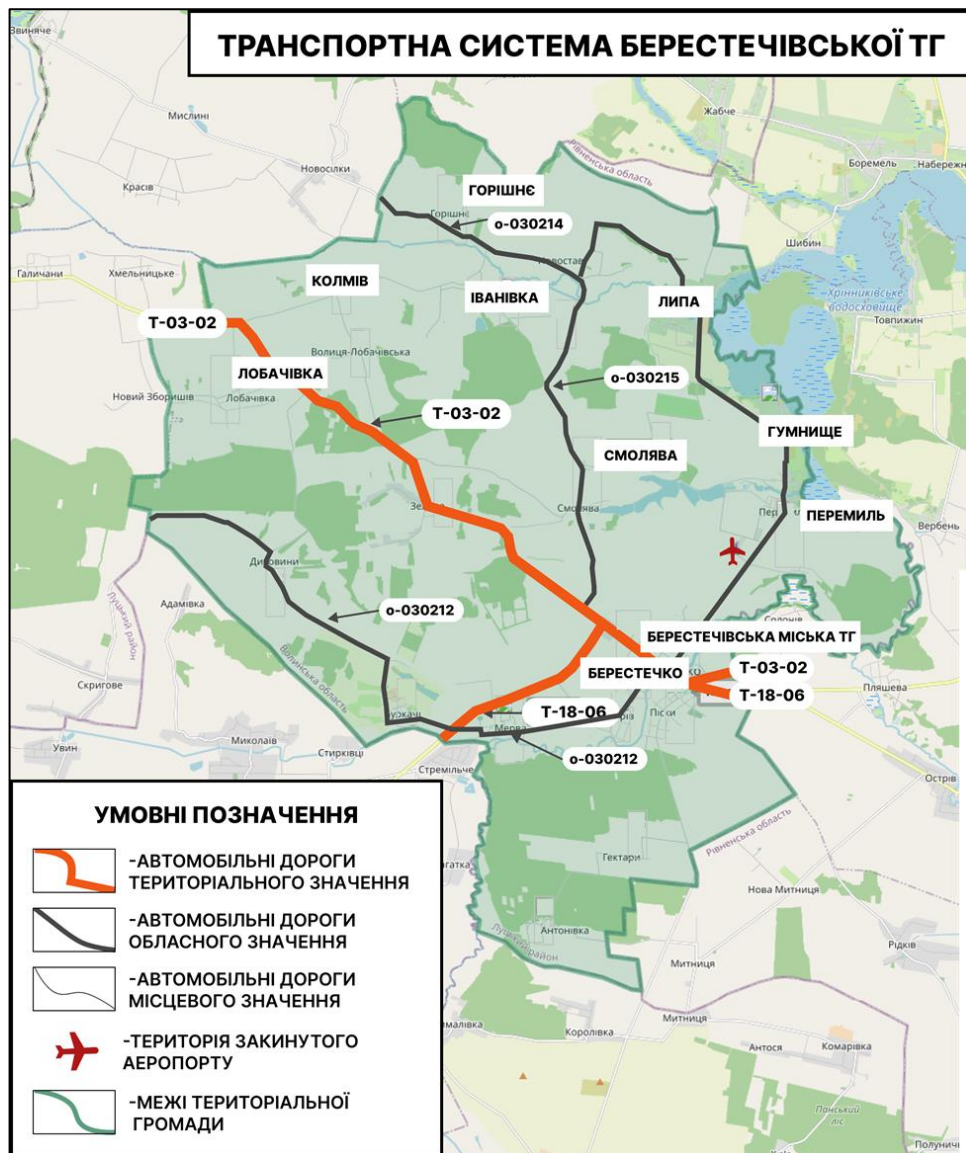
Рис. 2.9. Схема транспортної системи Берестечківської територіальної громади
