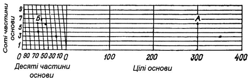
Рис. 4.5. Поперечний масштаб.
