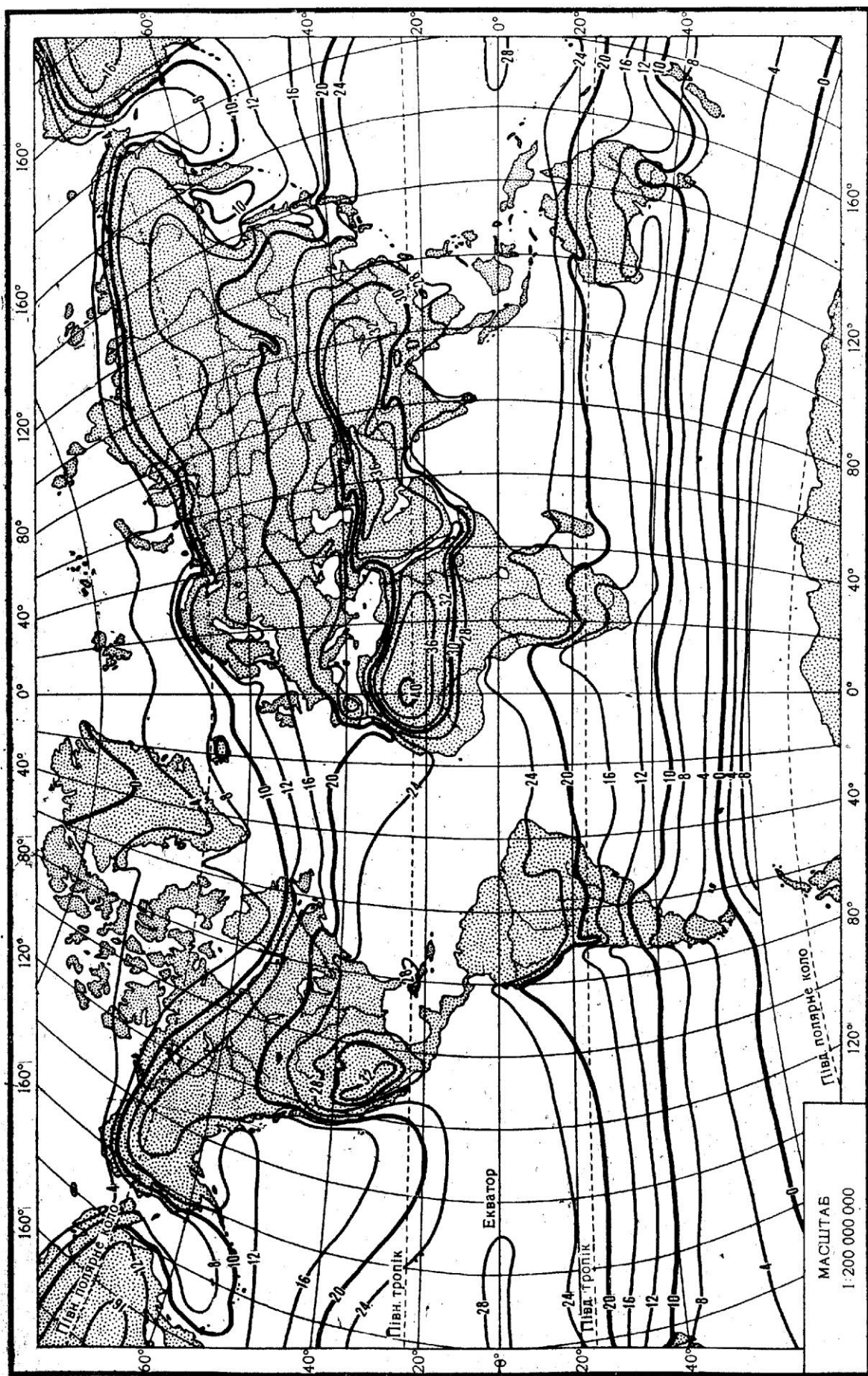
Рис. 10.2. Ізотерми липня.
