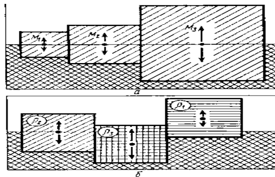
Рис. 1.2. Моделі ізостазії: а - за масою; б - за густиною речовини
