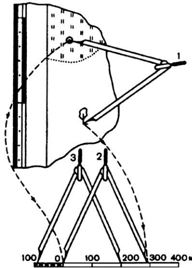
Рис. 4.4. Послідовність положень циркуля-вимірника під час знаходження відстані на карті за допомогою лінійного масштабу.
