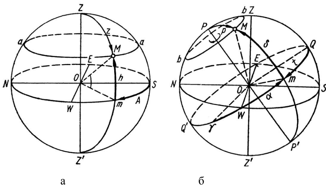
Рис. 3.1 Небесна сфера і системи координат:
