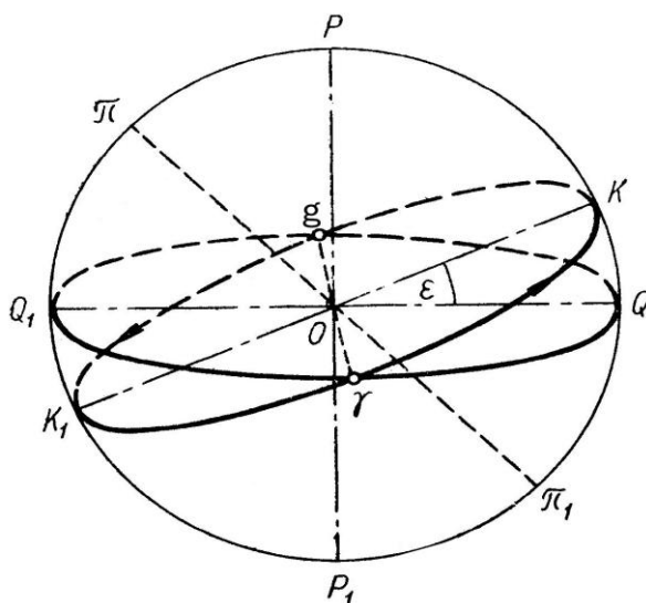
Рис. 3.2. Положення екліптики відносно небесного екватора.
