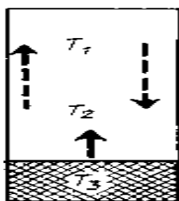
Рис. 1.6. Нестійкий стан повітря за умови адвекції тепла ззовні: тонкі лінії - ізобари, що утворюють «острів тепла».
