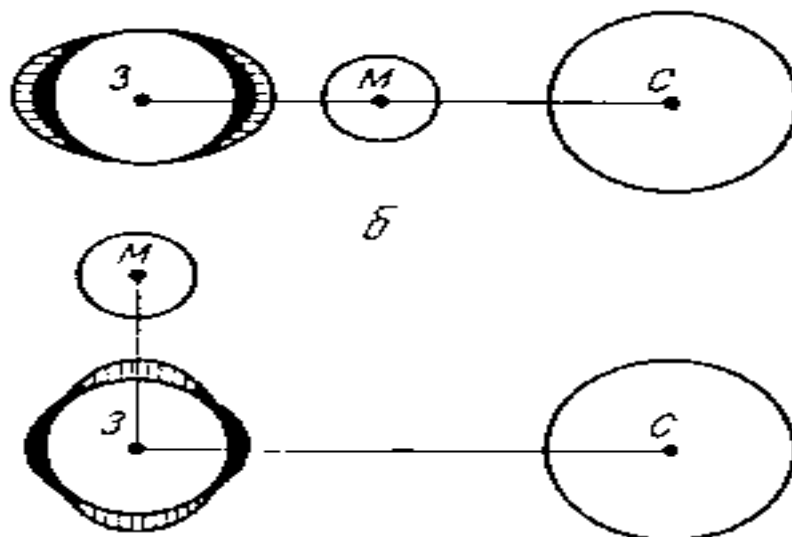
Рис. 1.4. Сизигійний (а, б) та квадратурний (в) припливи (З - Земля, М - Місяць, С - Сонце).
