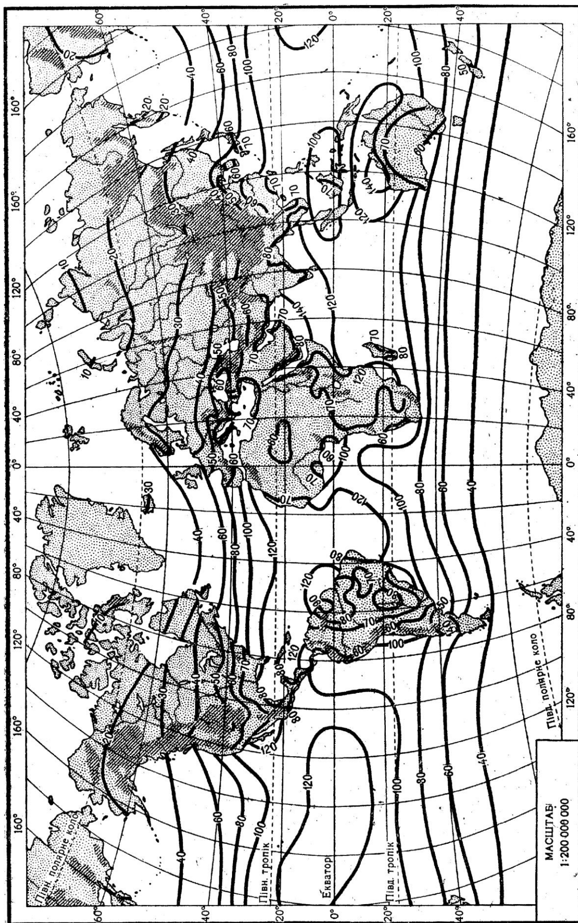
Рис. 9.3. Радіаційний баланс земної поверхні, ккал/(см 2 · рік).
