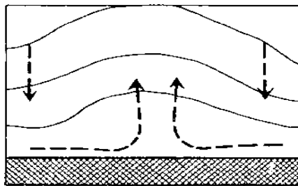
Рис. 1.5. Утворення термічної конвекції у нестійкому повітрі за умови нагрівання від земної поверхні: T_3 > T_2 > T_1 — - напрямок турбулентного теплопереносу та ----> - напрямок вертикальних потоків повітря.
