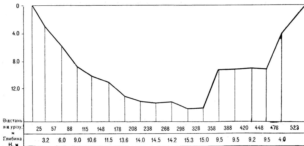
Рис. 16.2 Профіль поперечного перерізу озера Дальське по створу. I.
