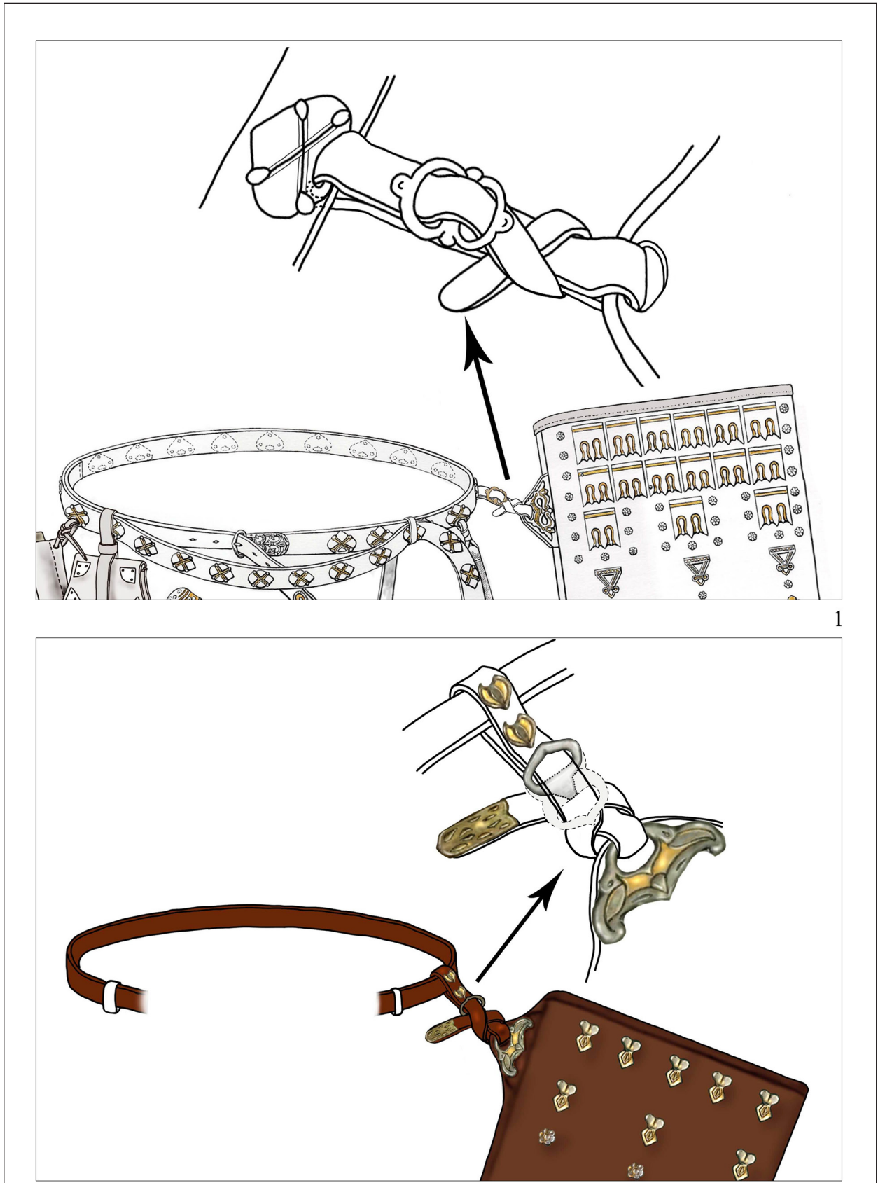
4. kép. A Karos-Eperjesszög III. temető 11. sír (1; Oleg Fjodorov nyomán) és a rovanci 5. sír (2) készenléti igtartótegez függesztésének rekonstrukciója
