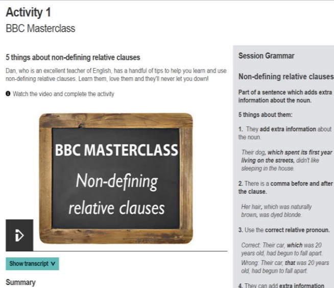
Рисунок 4. Розділ “BBCMasterclass”
